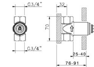
ZA 003330 Parte Incasso Rubinetto 3/4\"/>
