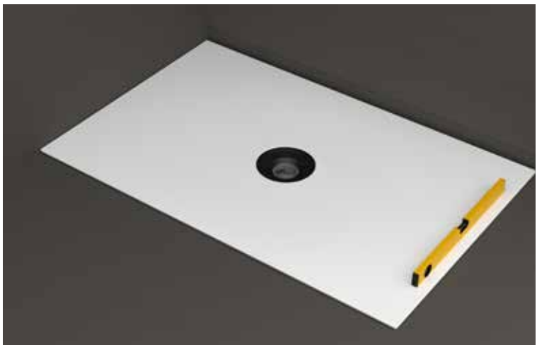
7 Установить плитку для душа
