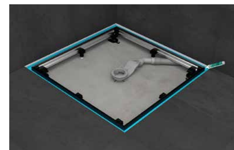
8 Точно установить гарнитуру
