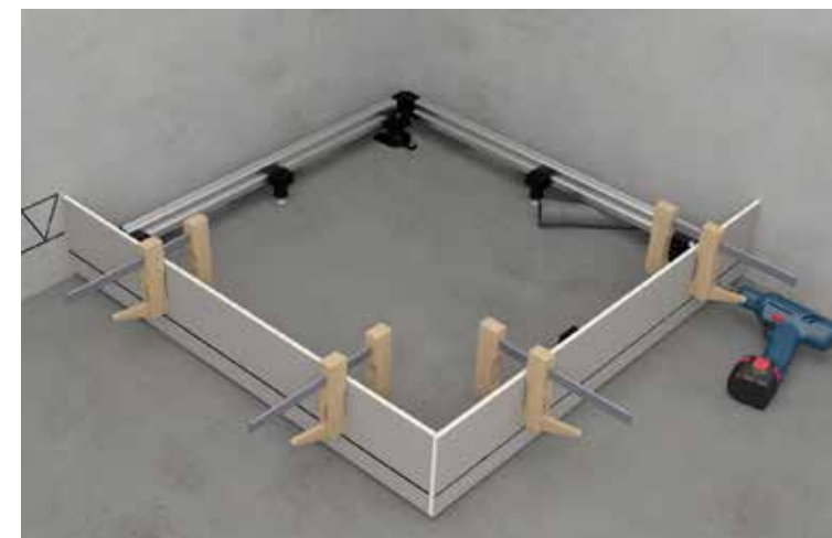
4 Смонтировать
