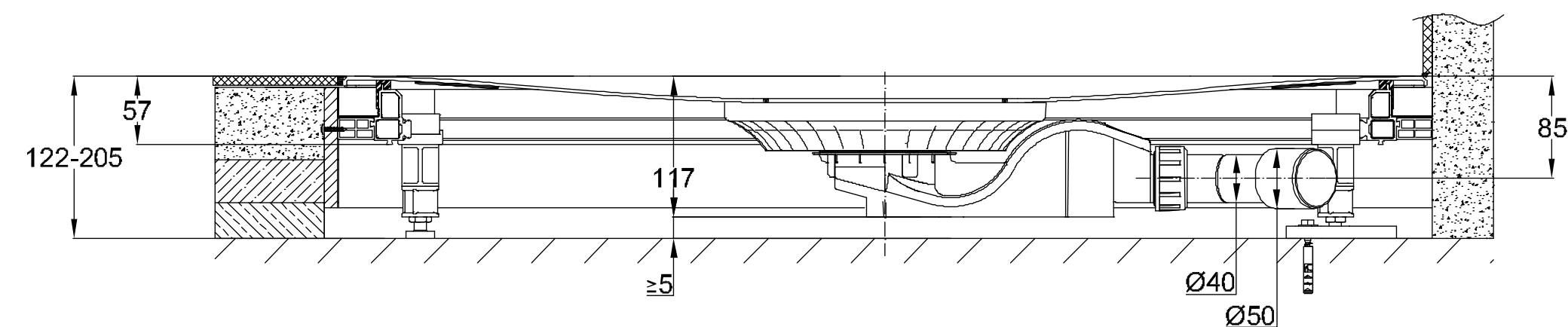
Рисунок монтажной системы Universal со сливной гарнитурой BetteAir 50 – 0,6 л/с, с боковым сливом, нормативный уровень воды в затворе 50 мм согл. EN 274
