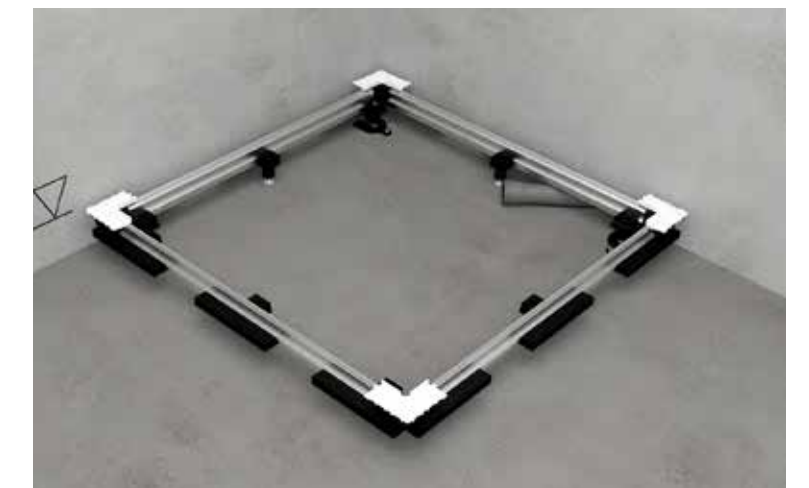
3 Расположить рамку
