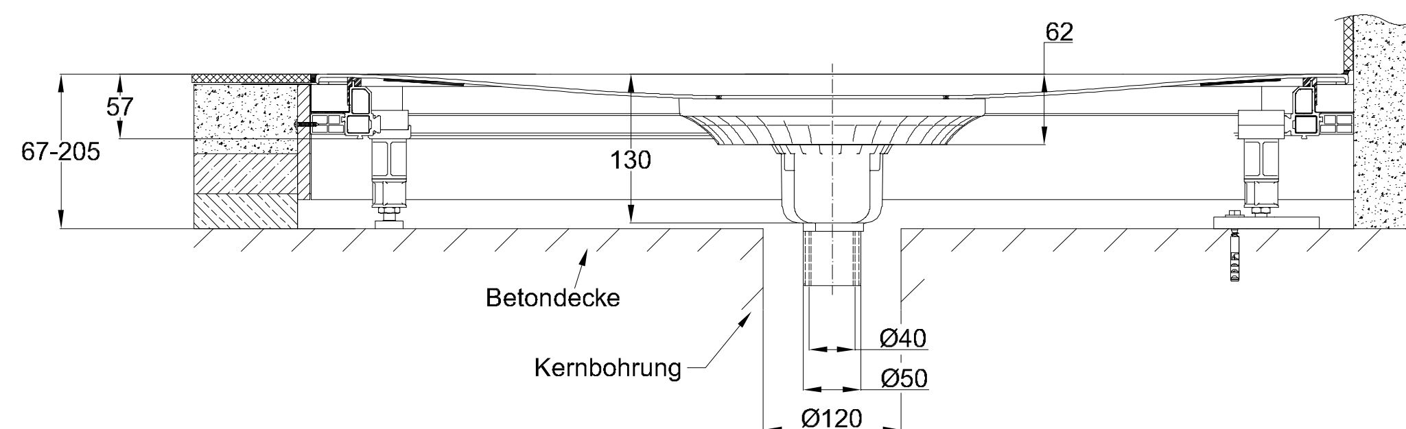
Рисунок монтажной системы Universal со сливной гарнитурой BetteAir Down 0,6 л/с, с боковым сливом, уровень воды в затворе 50 мм
